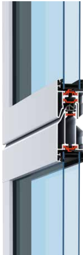
42 mm Thermo-Profil
