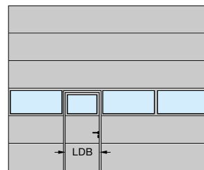
SPU F42, SPU 67 Thermo Alu-Verglasungsrahmen Schlupftüranordnung links
