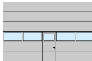
SPU F42, SPU 67 Thermo Alu-Verglasungsrahmen Schlupftüranordnung Mitte
